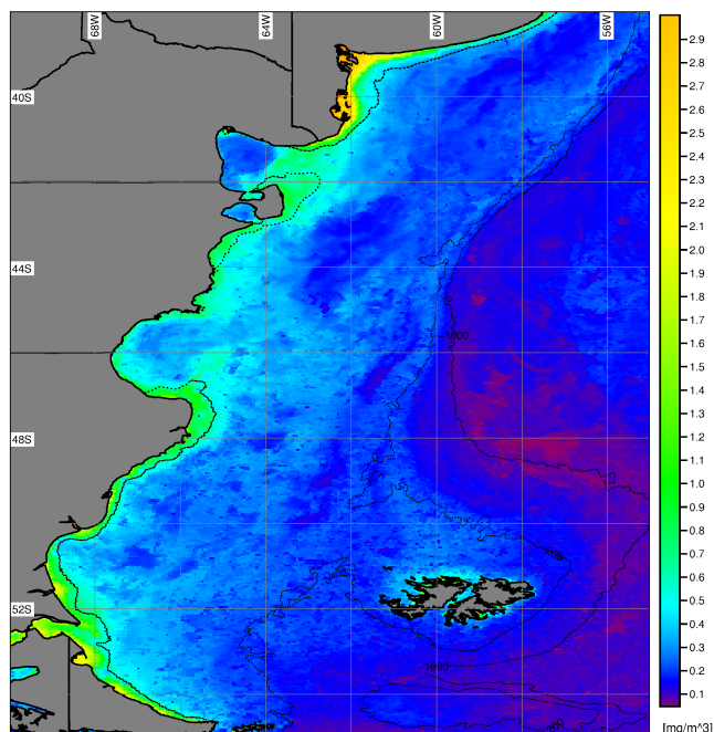
Figura B.3: Mínima de la concentración de clorofila ( \text{mg}/\text{m}^3 ) estimada a partir de MODIS/Aqua L3 en el período 2003-2013. Se muestran las isobatas de 200 y 1000 metros. La línea cercana a la costa representa el límite del área enmascarada a partir de la banda R_{rs}(667) (Sección 5.3.4.1).
