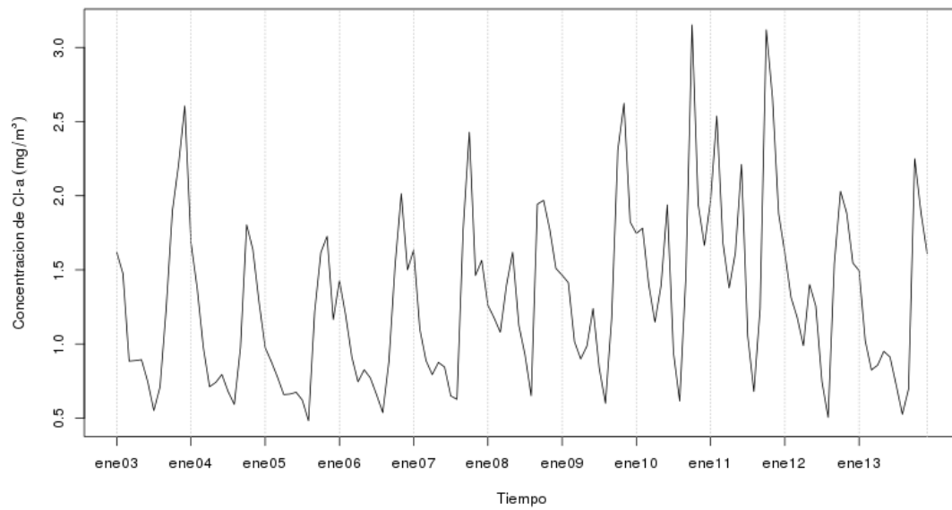
Figura 5.18: Serie de tiempo de la concentración media mensual de clorofila ( \text{mg}/\text{m}^3 ) estimada a partir de MODIS/Aqua L3 para el período 2003-2013 para toda el área de estudio.
