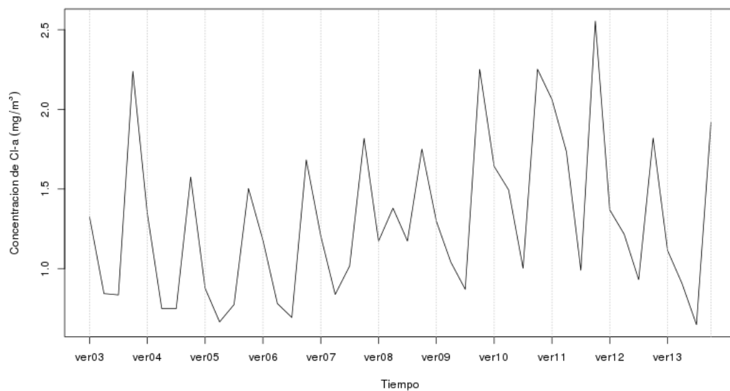
Figura 5.19: Serie de tiempo de la concentración media estacional de clorofila ( \text{mg}/\text{m}^3 ) estimada a partir de MODIS/Aqua L3 para el período 2003-2013 para toda el área de estudio.
