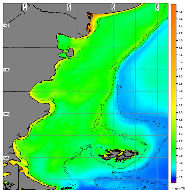
Figura B.1: Mediana de la concentración de clorofila ( \text{mg/m}^3 ) estimada a partir de MODIS/Aqua L3 en el período 2003-2013. Se muestran las isobatas de 200 y 1000 metros. La línea cercana a la costa representa el límite del área enmascarada a partir de la banda R_{rs}(667) (Sección 5.3.4.1).
