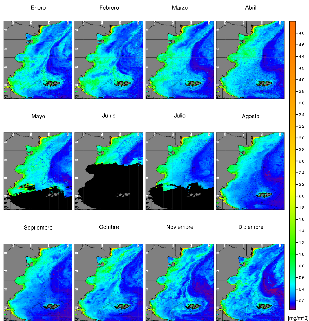
Figura B.25: Moda mensual de la concentración de clorofila ( \text{mg}/\text{m}^3 ) estimada a partir de MODIS/Aqua L3 en el período 2003-2013. Zonas en negro representan áreas sin datos. Se muestran las isobatas de 200 y 1000 metros. La línea cercana a la costa representa el límite del área enmascarada a partir de la banda R_{rs}(667) (Sección 5.3.4.1).
