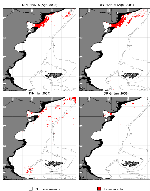
Figura 6.21: Área mínima con concentraciones de Cl-a mayores a 1.05 \times \text{mediana} . Se muestran las isobatas de 200 y 1000 metros. La zona en negro representa el área enmascarada a partir de la banda R_{rs}(667) (Capítulo 5, Sección 5.3.4.1).
