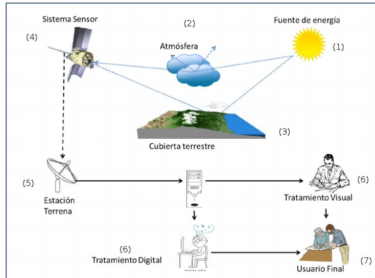
Figura 2.3: Componentes de un sistema de teledetección (Chuvieco, 2010).
