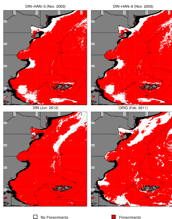
Figura 6.20: Área máxima con concentraciones de Cl-a mayores a 1.05 \times \text{mediana} . Se muestran las isobatas de 200 y 1000 metros. La zona en negro representa el área enmascarada a partir de la banda R_{rs}(667) (Capítulo 5, Sección 5.3.4.1).
