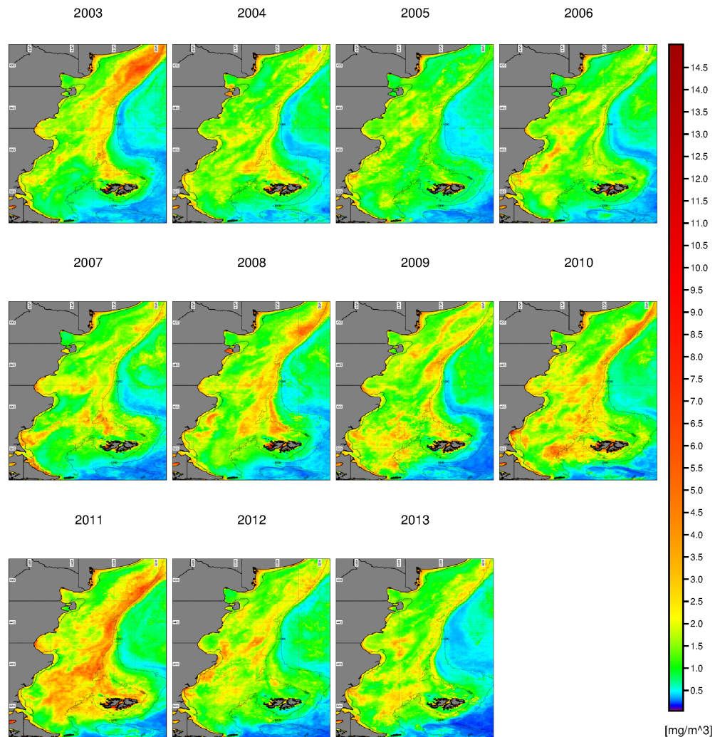
Figura 5.7: Media anual de la concentración de clorofila ( \text{mg/m}^3 ) estimada a partir de MODIS/Aqua L3 en el período 2003-2013. Se muestran las isobatas de 200 y 1000 metros. La línea cercana a la costa representa el límite del área enmascarada a partir de la banda R_{rs}(667) (Sección 5.3.4.1).
